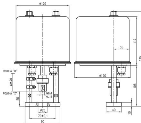
připojení P2 - příruba na Ø 25, spojka M8x1
