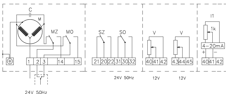
tříbodové řízení - 24 V, 50Hz
