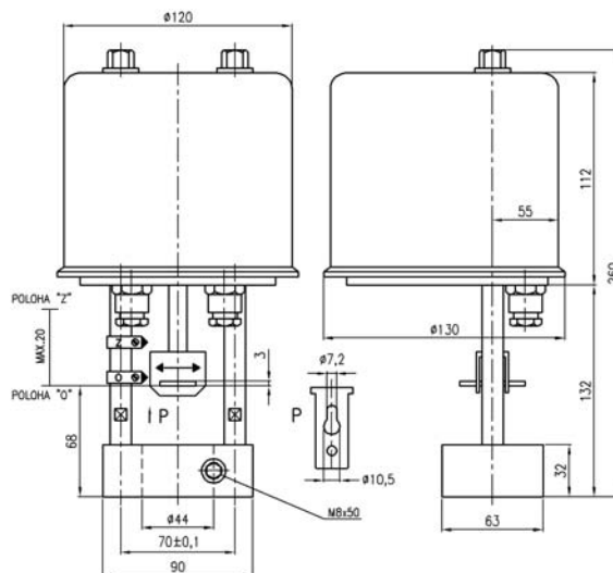
připojení P3 - příruba na Ø 44, vřeteno se zářezem
